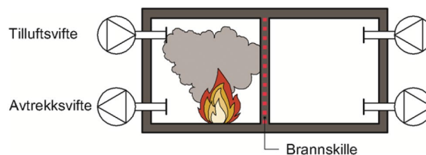
Figur 3-1 Prinsippkisse som viser løsningen med å benytte separate ventilasjonsanlegg i hver branncelle. Illustrasjon: Bygghetjserien 520.352, SINTEF Bygghetj [9].
