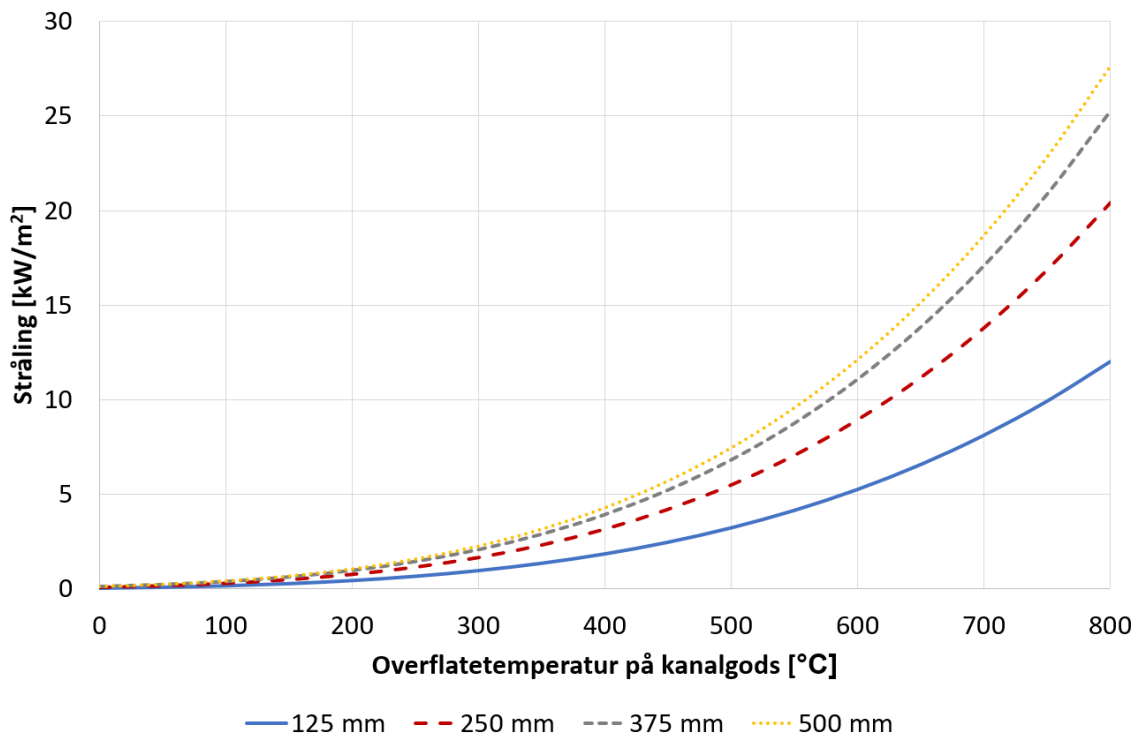
Figur 2-11 Stråling på materialelement normalt på uisolert kanal. I beregningene er det benyttet en emissivitet lik 0,8 og en avstand på 25 cm som gir synsfaktor 0,20 , 0,33 , 0,43 og 0,50 for henholdsvis 125 mm, 250 mm, 375 mm og 500 mm kanal.
