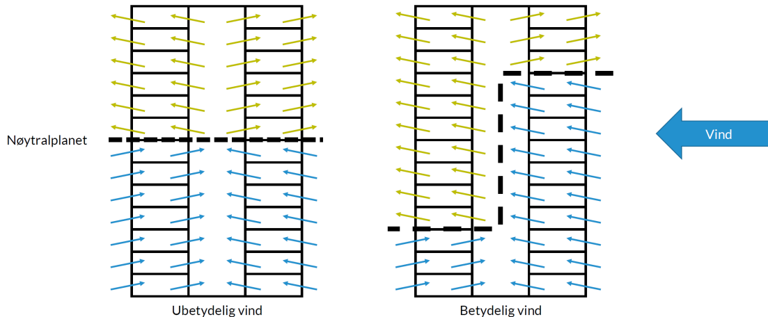
Figur 2-18: Innflytelsen av vinden på luftbevegelsene i et høyt bygg, samt hvordan nøytralplanet (stiplet linje) forandrer seg som følge av vinden. Figuren er basert på [23].
