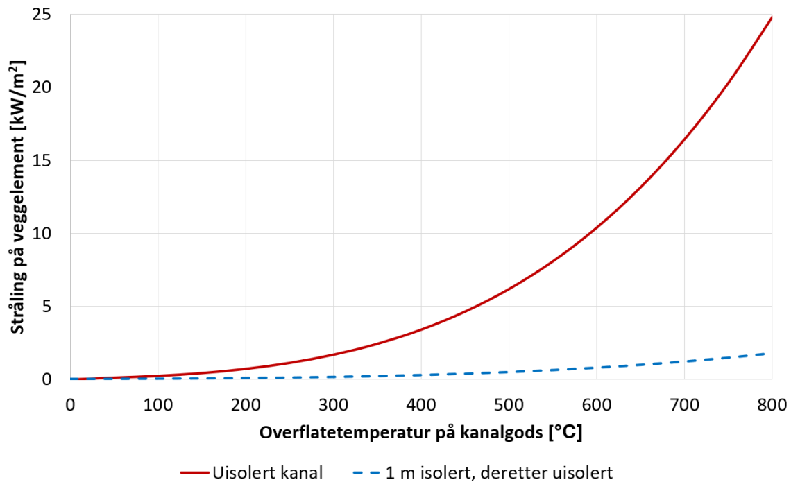
Figur 2-6 Strålingsnivå på et vegglement der kanalen er uisolert og der kanalen har den første meteren isolert, deretter uisolert. Det er benyttet en synsfaktor på 0,5 og 0,03 for henholdsvis uisolert og isolert kanal. Emissiviteten er for begge tilfeller lik \epsilon = 0,8 .
