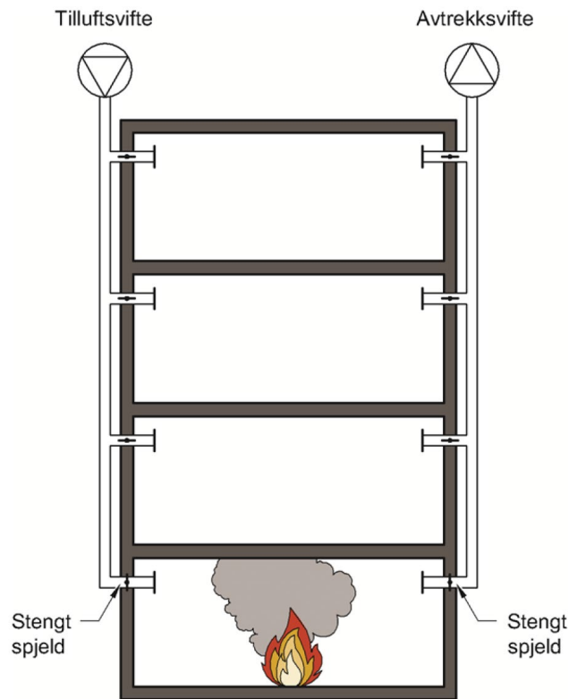
Figur 3-2 Prinsippskisse som viser steng-inne-løsningen. Spjeld på tilluftskanal og avtrekkskanal stenges for å stenge røyk og varme inne i branncellen. Illustrasjon: Byggforskserien 520.352, SINTEF Byggforsk [9].
